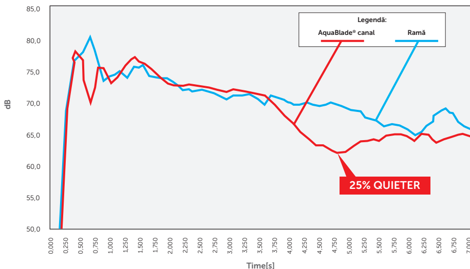
dB Graficul zgomotului în funcție de tipul vasului wc.
